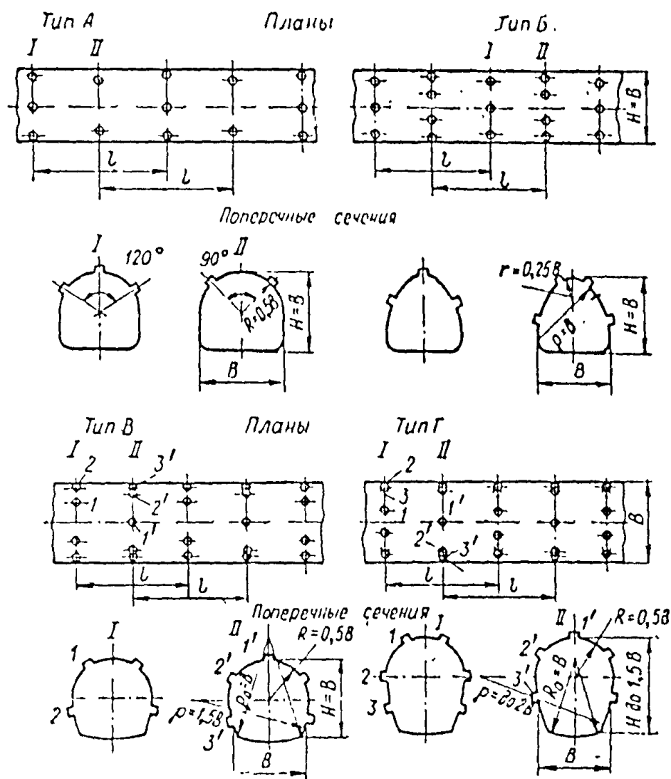
Рис. 1. Схемы расположения цементационных скважин
