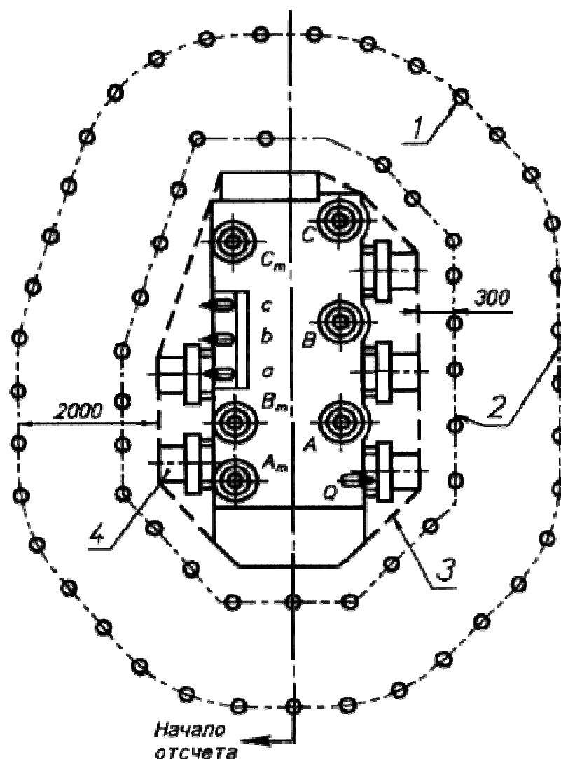
1 - микрофон; 2 - измерительная линия; 3 - излучающая поверхность; 4 - охладитель
